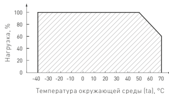
Рис. 3. Максимальная допустимая нагрузка, % от мощности источника.
